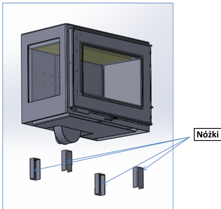
Ilustracja 11 Sytuacja nóżek i ich śrubek
