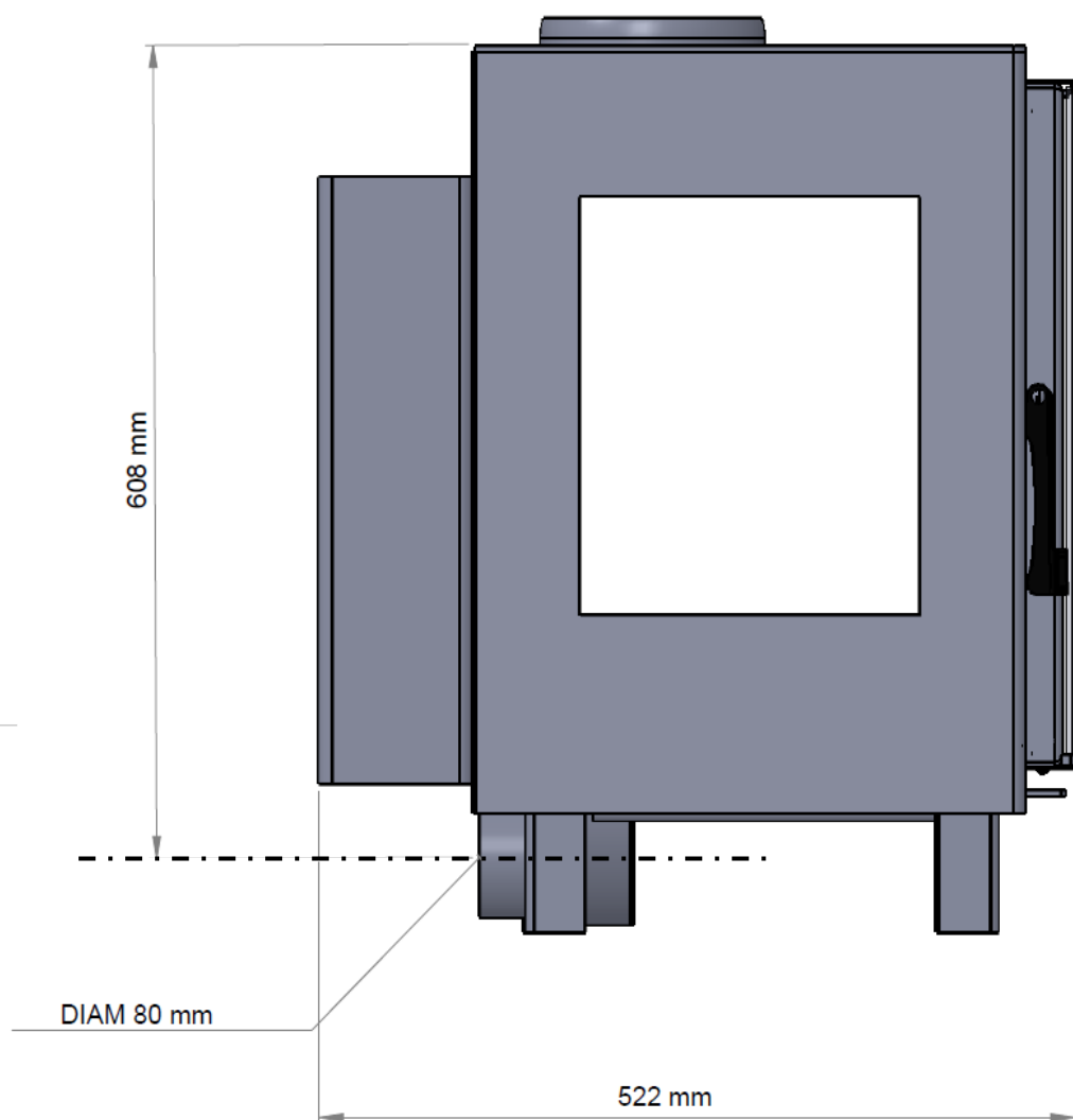
Illustration1. Plan général
