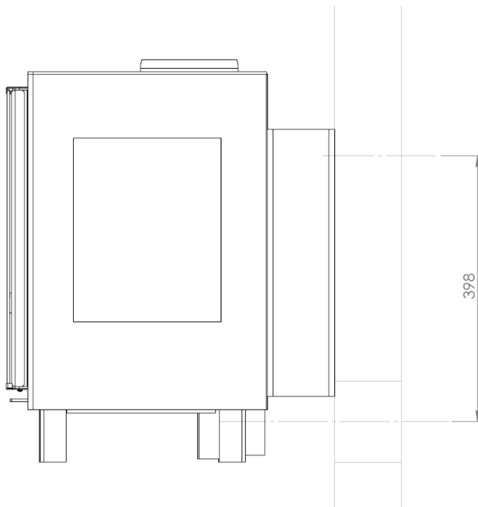
Ilustracja 4. Rysunek dołotu powietrza z zewnątrz
