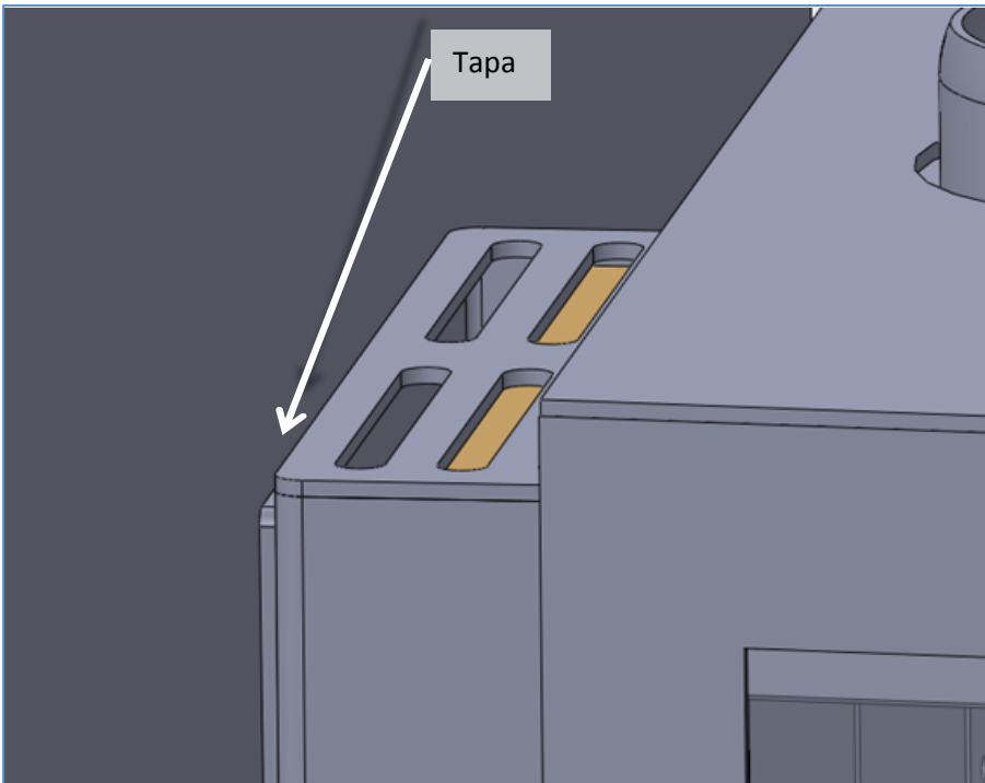
Ilustración 10. Colocación tapa
