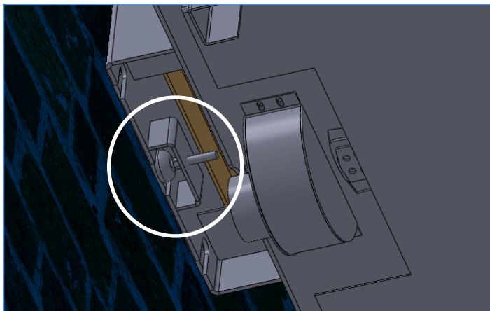
Ilustracja 7. Sytuowanie regulatora.
