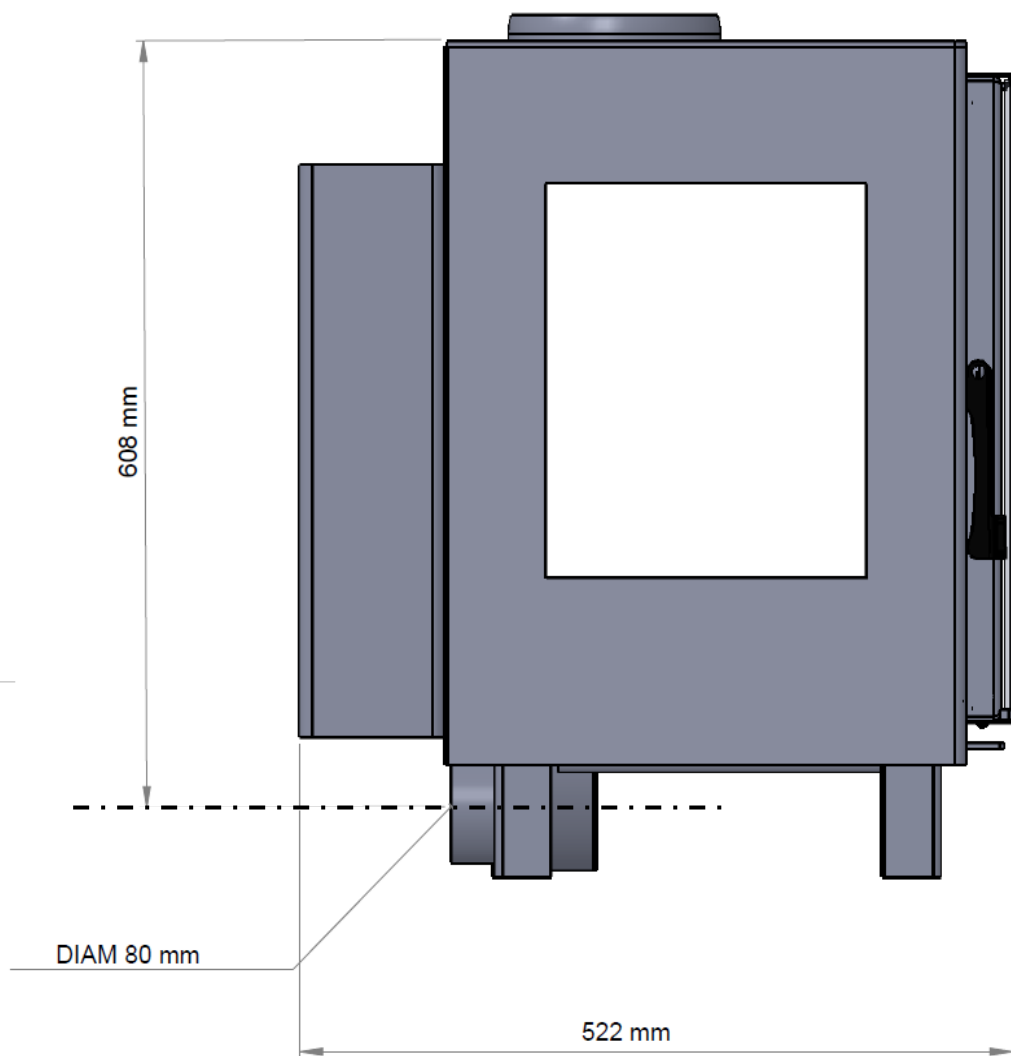
Ilustracja 1. Krysunek główny
